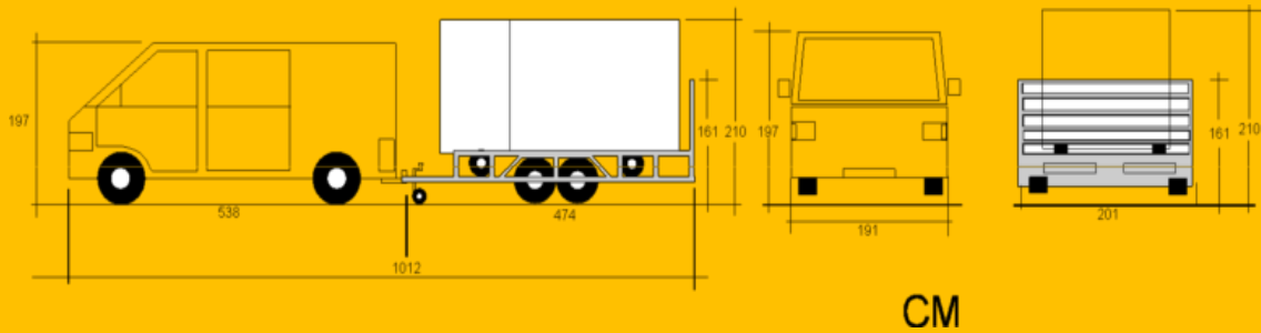
Croquis del vehicle de transporte del Drago:
